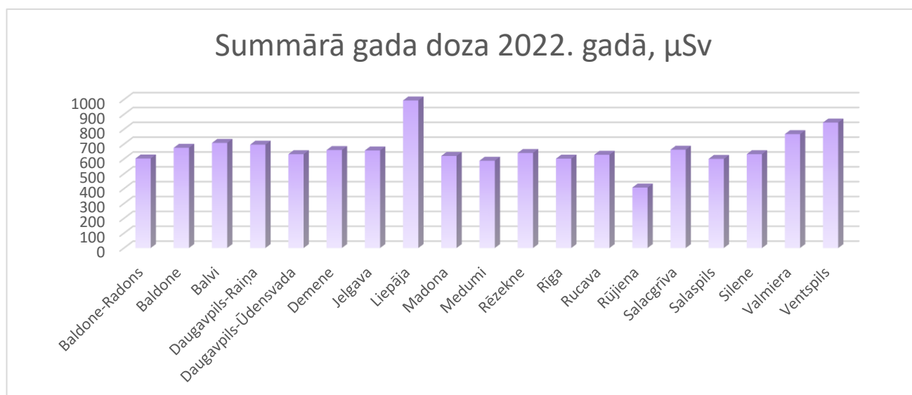
1.attēls. Summārās gada gamma dozas, 2022. gads
