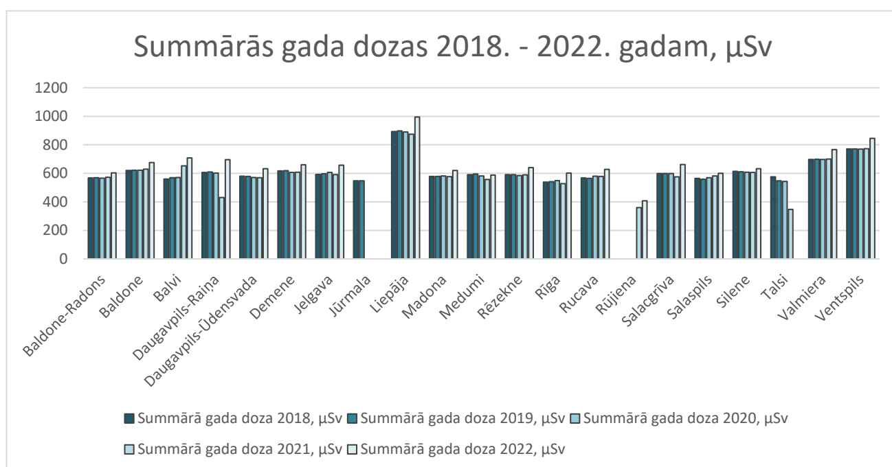
2.attēls. Summārās gada gamma dozas no 2018. līdz 2022. gadam
