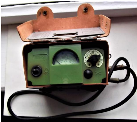
35.attēls. Izplatītākās radiometra DP-5 modifikācijas Latvijā (DP-5A un DP-5B)
